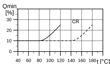
Fig. 17 Débit mini
