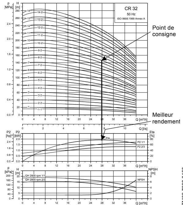
Fig. 9 Exemple d'un point de consigne d'une pompe CR
