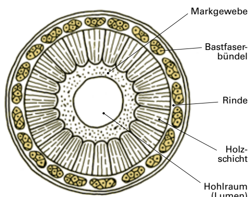
3 Flachsstengelquerschnitt, schematisch
